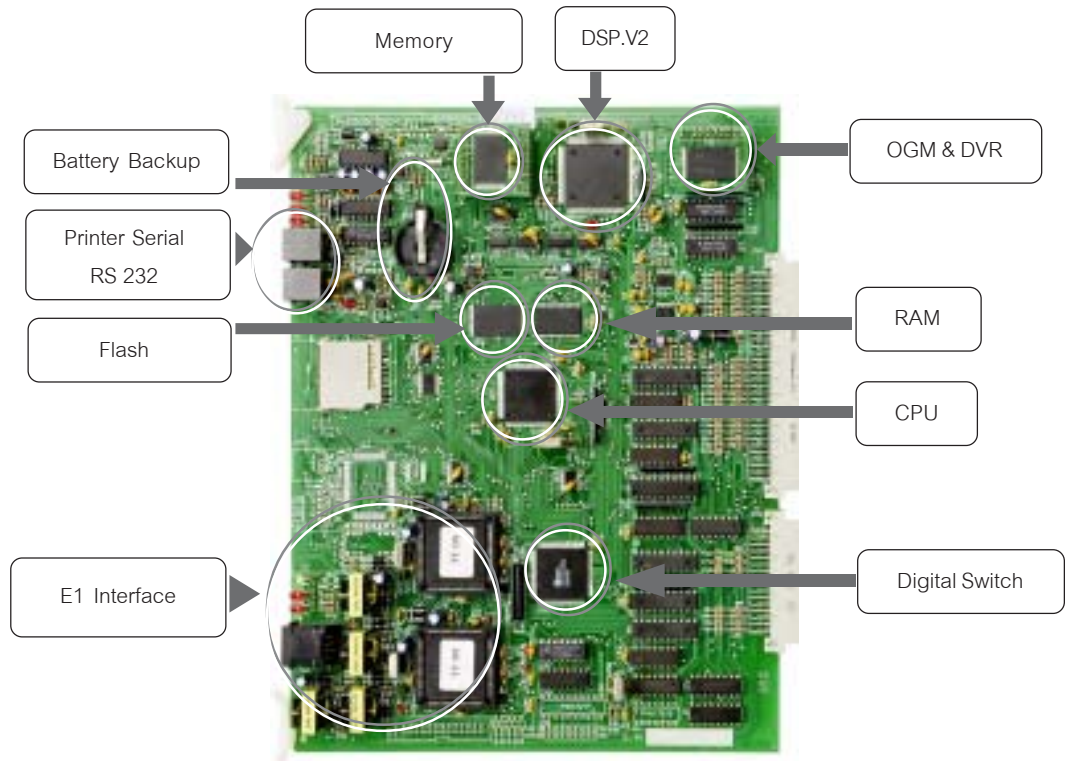
รูปที่ 4.1 แสดงการวางอุปกรณ์ของแผง DX-LPU/PRI.V3
