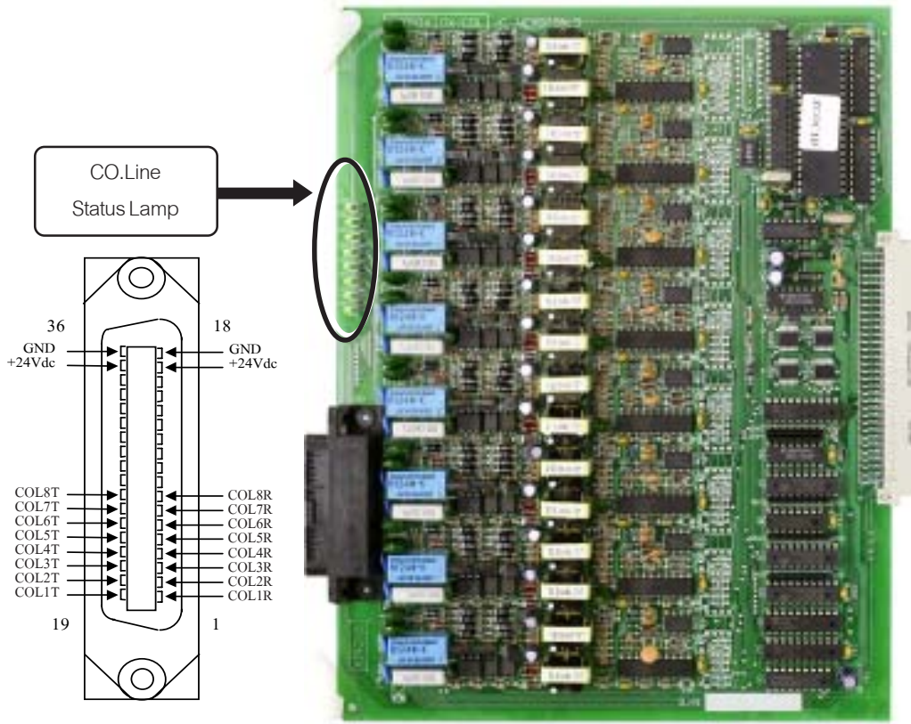
รูปที่ 4.3 แสดงการวางอุปกรณ์ของแผง DX-8COL/C.V3
