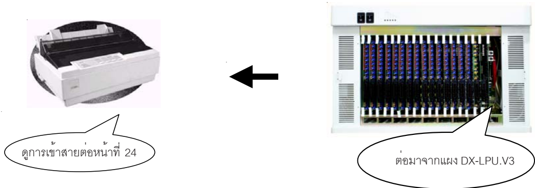
รูปที่ 7.6 แสดงการต่อ Printer
