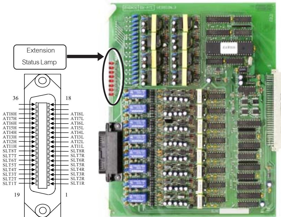
รูปที่ 4.5 แสดงการวางอุปกรณ์ของแผง DX-8ATI.V3
