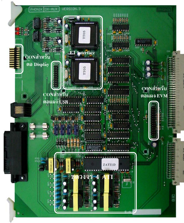
รูปที่ 4.2 แสดงการวางอุปกรณ์ของแผง DX-AUX/PRI.V3
