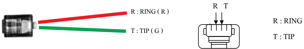
รูปที่ 10.2 แสดงการเข้าสายของเครื่อง DSS
