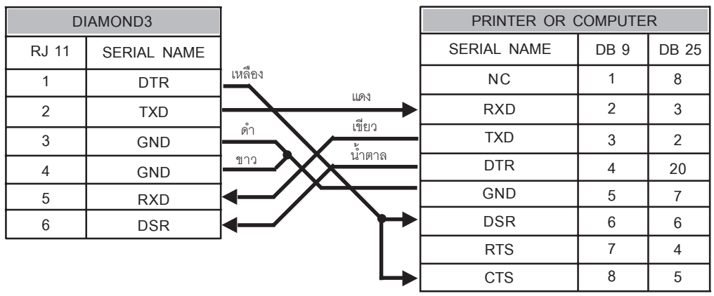
รูปที่ 11.3 แสดงการต่อสายสัญญาณ Serial RS-232
