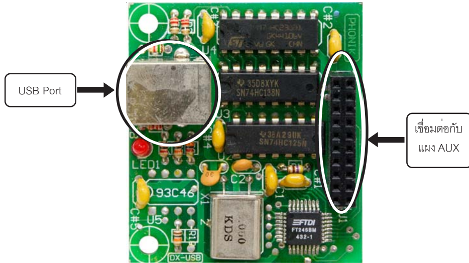
รูปที่ 5.2 แสดงการวางอุปกรณ์ของแผงรุ่น USB
