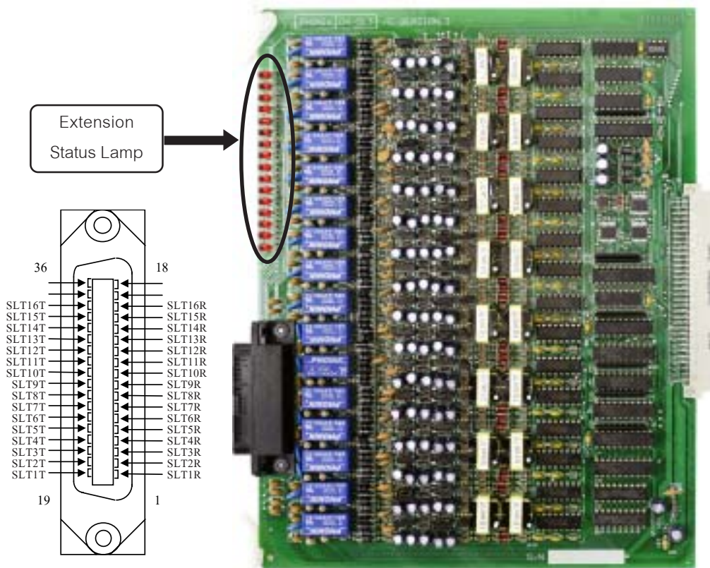
รูปที่ 4.4 แสดงการวางอุปกรณ์ของแผง DX-16SLT/C.V3
