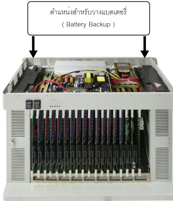
รูปที่ 6.5 แสดงตำแหน่งการต่อ Battery Backup
